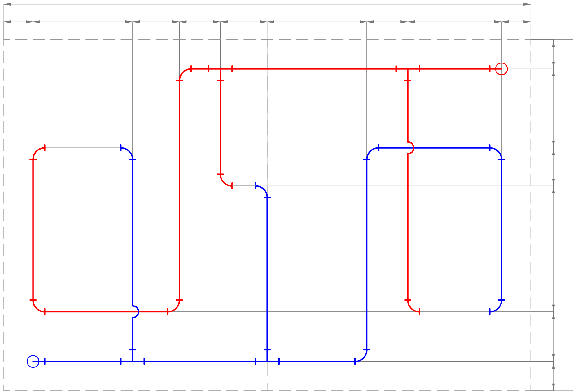
NATJECANJE VODOINSTALATERA 2017. ZADATAK B - RAZVOD VODE MAT.: PP-R: 20x3.4
