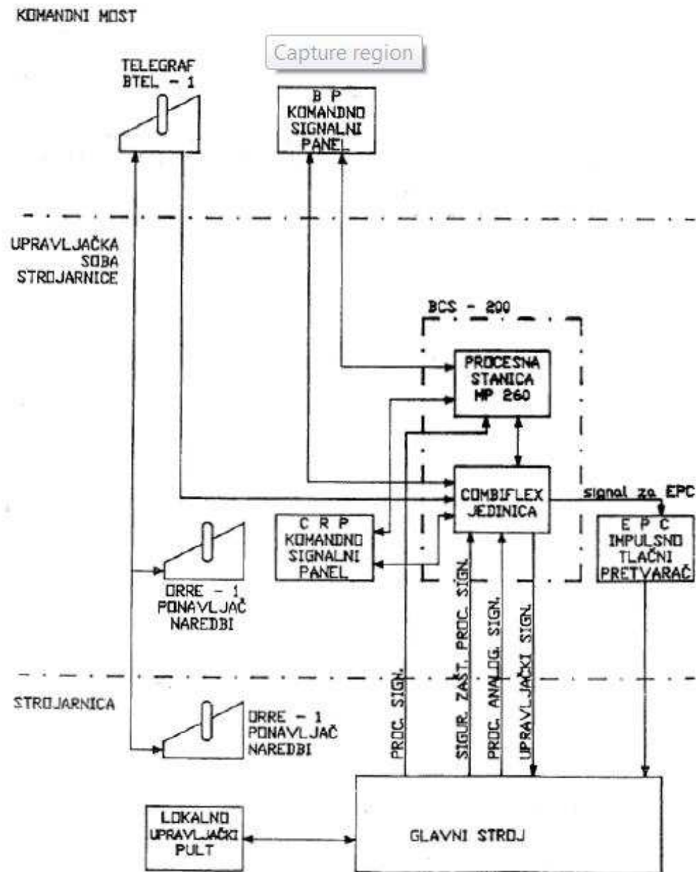
Slika 2.1 Strukturna blok shema sustava BCS 200
